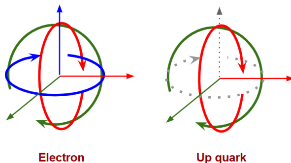
図3-5. アップクォークの2つの回転ベクトル
